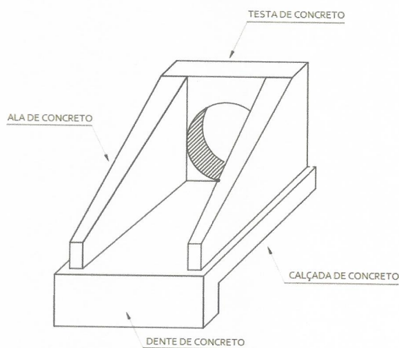
Figura 11 - Boca de bueiro tubular de concreto
