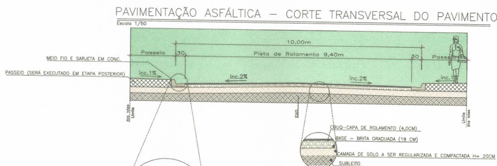
Figura 14 - Corte transversal no pavimento
