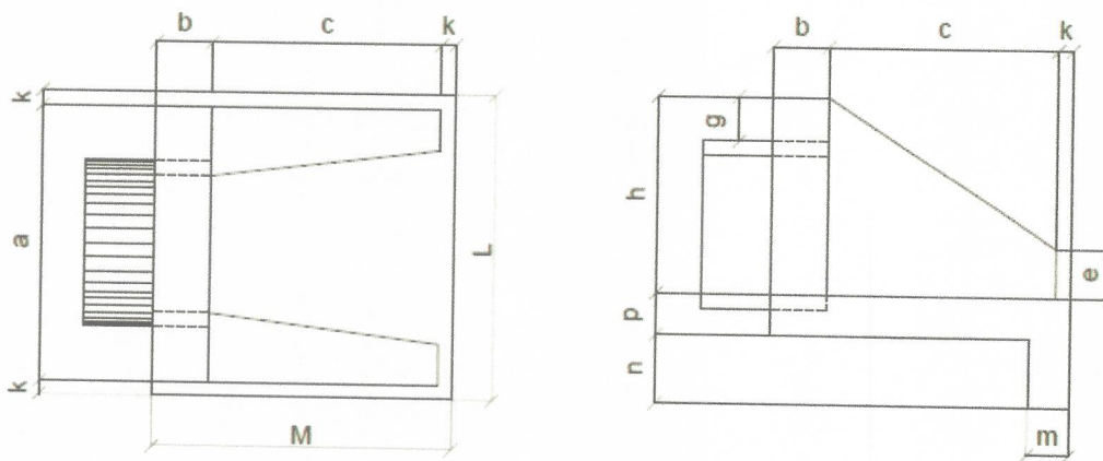
Figura 13 - Vistas superior e lateral da boca de bueiro simples tubular
